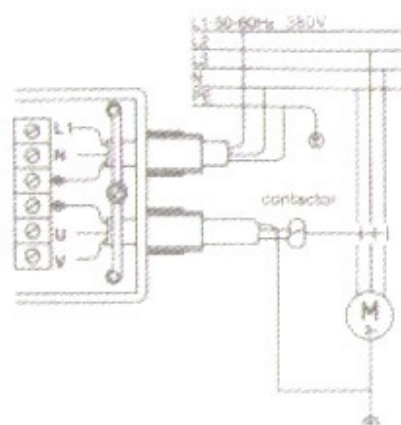
Під'єднання насосів потужністю більш ніж 1.1кВт 380В через вимикач
